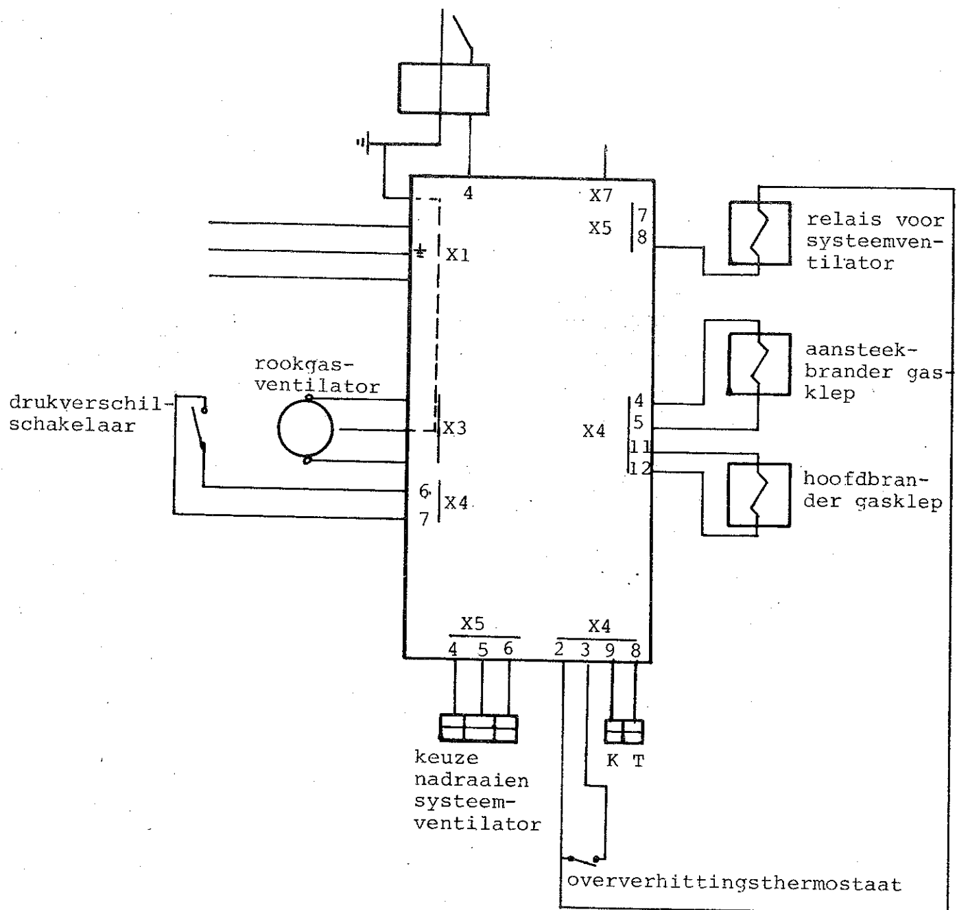
Figuur 8 : Aansluitschema besturingskast Philips MCBA 0211.
