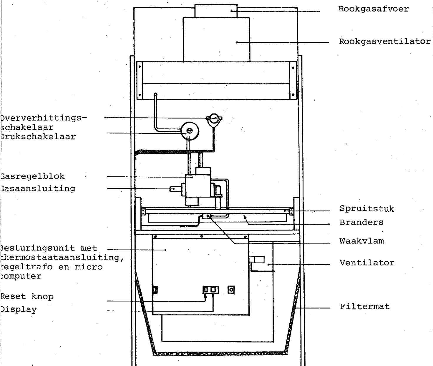
Figuur 6 :Vooraanzicht luchtverwarmer type H met bedieningsapparatuur.
